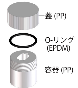
※4: S2400 Li箔保存容器
